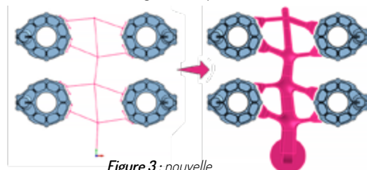
Figure 3 : nouvelle conception du système de remplissage
