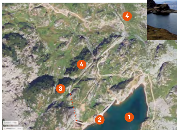
(6) prise d'eau ancienne sous le lac Crozet. (D) Vue aérienne du lac Crozet (1) : barrage (2), prise d'eau (3), conduite forcée installée par les Papeteries de France en 1956 (4) - Source Géoportail, prise de vue 2024
