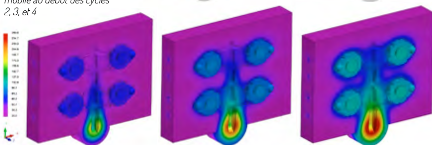
Figure 8 : champ de température dans le moule mobile au début des cycles 2, 3, et 4
