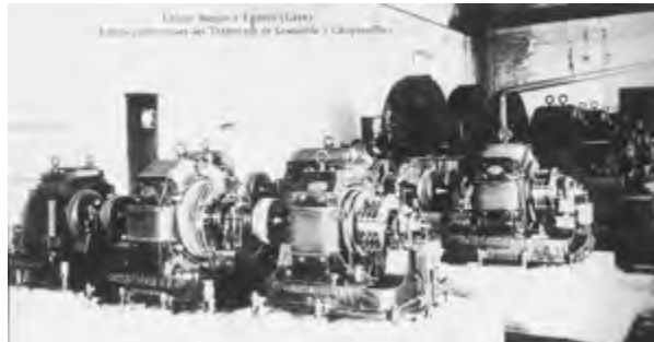
Centrale à Lancey. Forces génératrices des Tramways de Grenoble à Chapareillan
